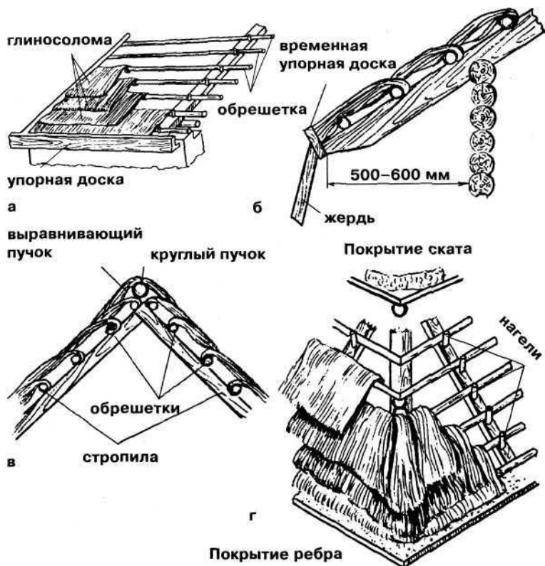
Рис. 23. Глиносоломная кровля
