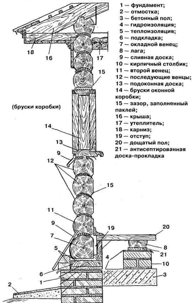
Рис. 46. Устройство стены бревенчатой бани
